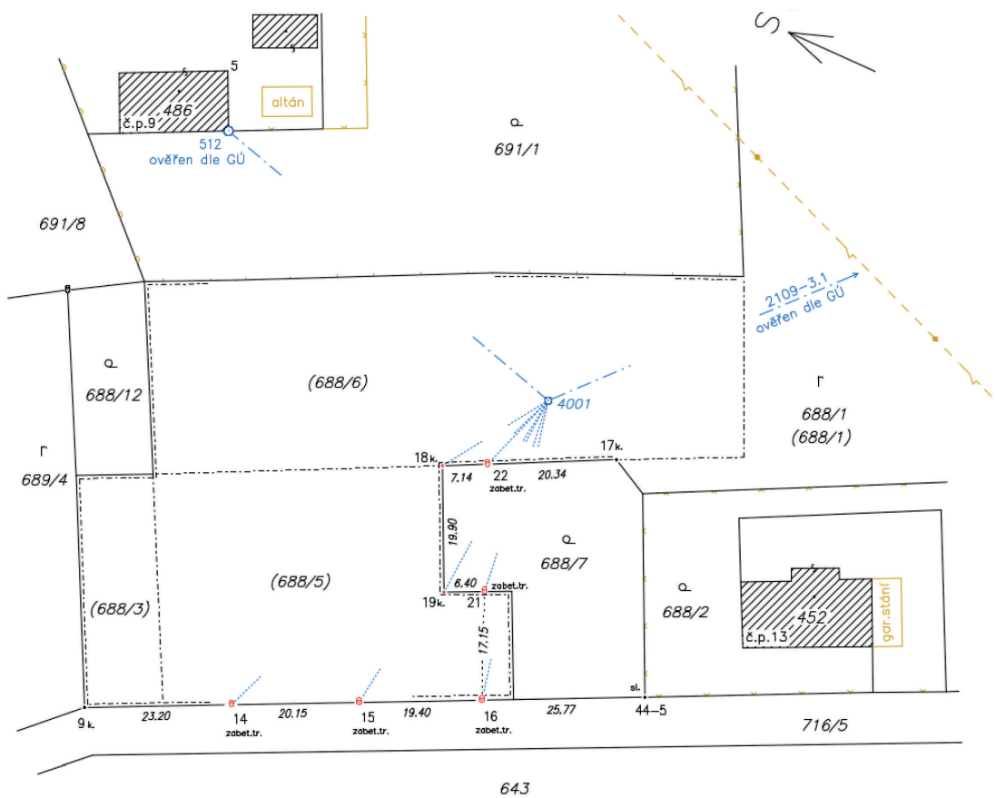
„16.28 Vzor vytyčovacího náčrtu
